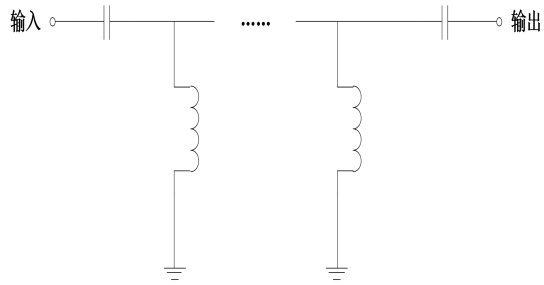
YLLP-1100-D4-W7.8产品原理图
